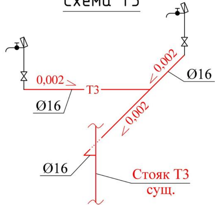
Схема Т3
